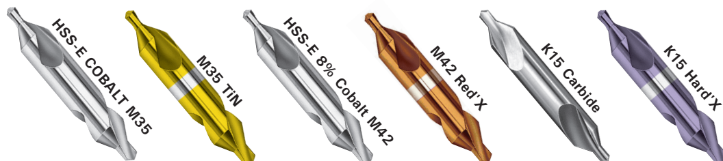
Plain Center Drills - Angle 60° ISO - NFE 66051-A - DIN 333-A - JIS-1
