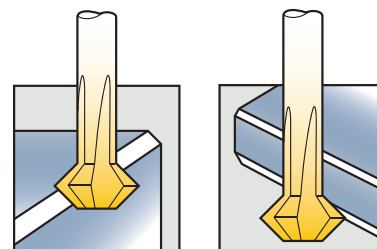
Top Chamfering
