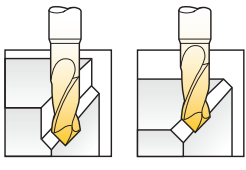
60°-90°-120° Longitudinal Chamfers
