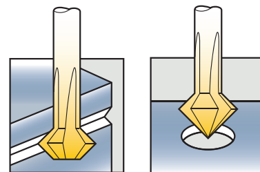
V-Grooving
